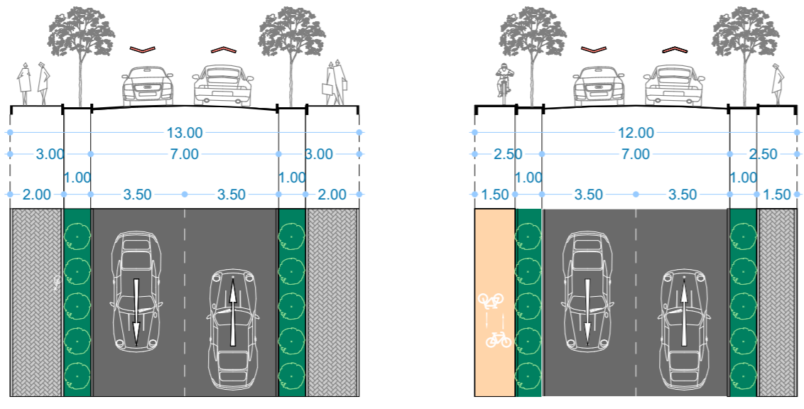
PROFIL PROPUS S-01 conf. P.U.Z. Centru cultural Șumuleu aprobat prin H.C.L. nr. 175/2014
